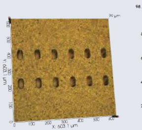
금도금 마이크로비아
